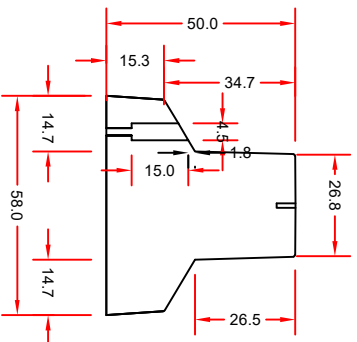
SEZ. D-D
