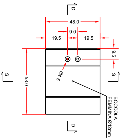
PIANTA
